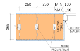
- VÄZBA PŘI DVEROVOM OSTĚNÍ, 2. RADA MURIVA
