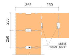
- VÄZBA ROHU, 1. RADA MURIVA
