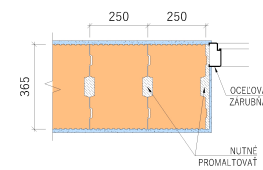
- VÄZBA PŘI DVEROVOM OSTĚNÍ, 1. RADA MURIVA
