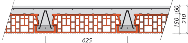
Hrúbka stropu 210 mm - max. dĺžka stropného nosníka 6 250 mm
