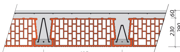
Hrúbka stropu 290 mm
