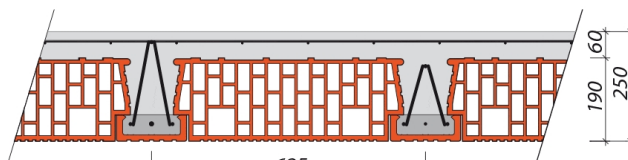
Hrúbka stropu 250 mm
