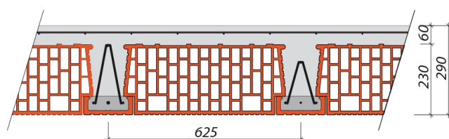
Hrúbka stropu 290 mm
