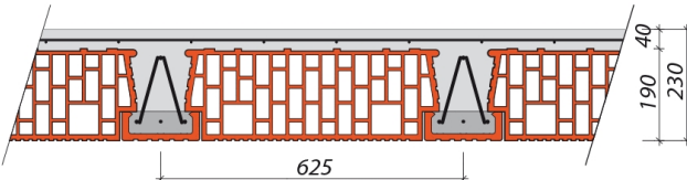
Hrúbka stropu 230 mm - max. dĺžka stropného nosníka 6 250 mm
