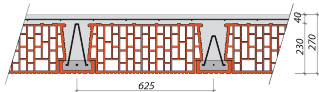
Hrúbka stropu 270 mm
