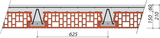
Hrúbka stropu 210 mm - max. dĺžka stropného nosníka 6 250 mm
