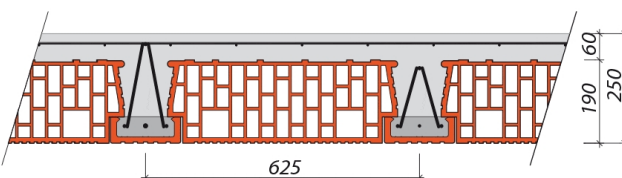
Hrúbka stropu 250 mm
