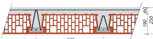
Hrúbka stropu 250 mm
