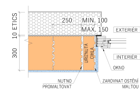
- VAZBA U OKENNÍHO OSTĚNÍ, 2. ŘADA ZDIVA
