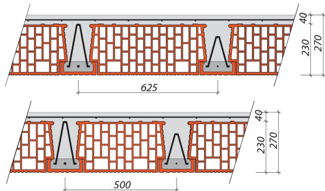
Hrúbka stropu 270 mm
