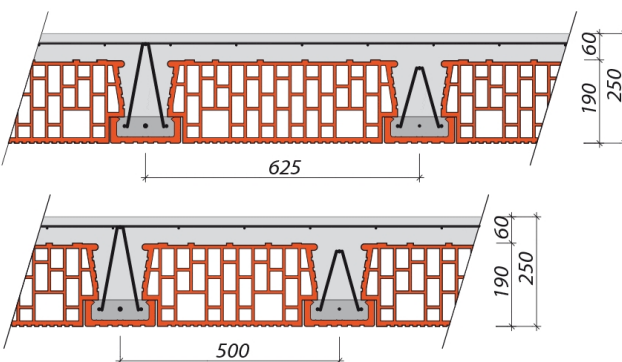
Hrúbka stropu 250 mm
