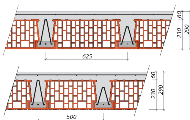
Hrúbka stropu 290 mm
